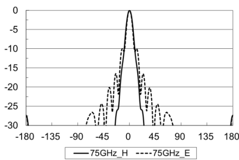
75GHz
