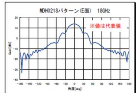
18GHz(E面)
