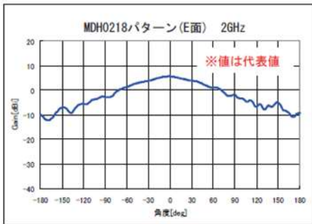
2GHz(E面)
