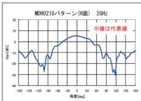
2GHz(H面)
