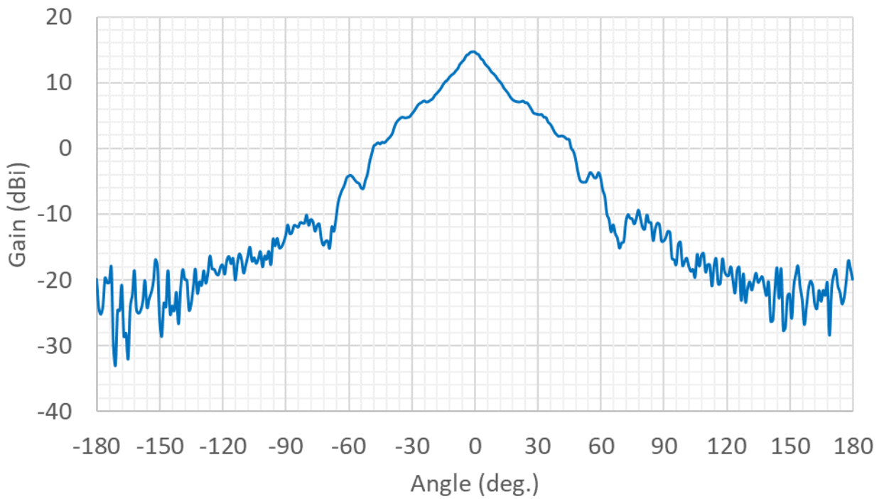
18GHz (E面)
