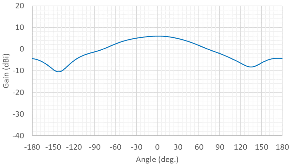
1GHz (E面)
