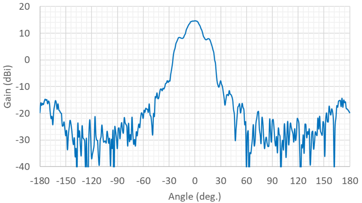
18GHz (H面)
