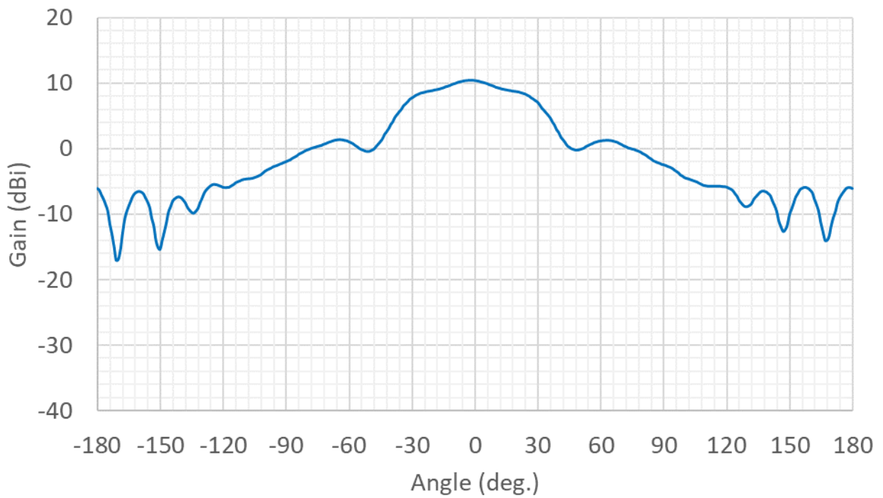
5GHz (E面)
