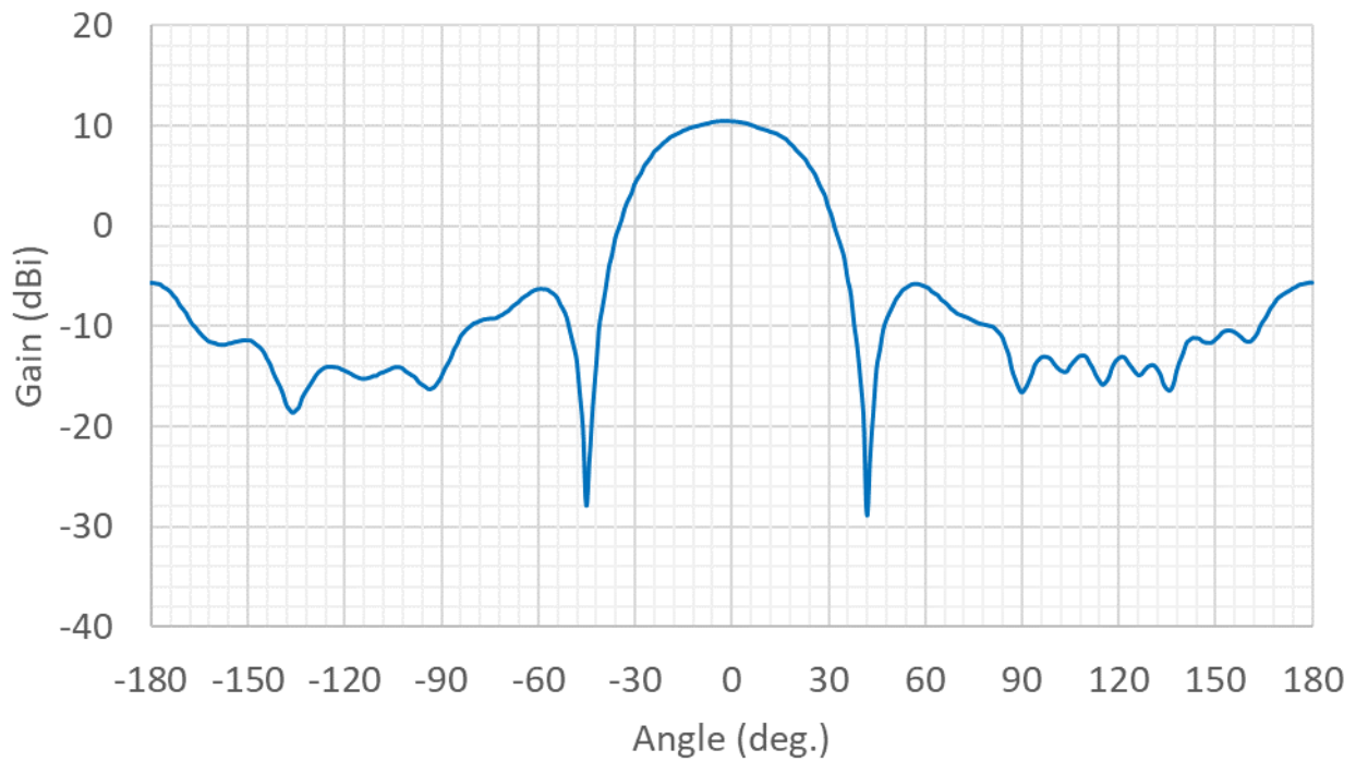
5GHz (H面)
