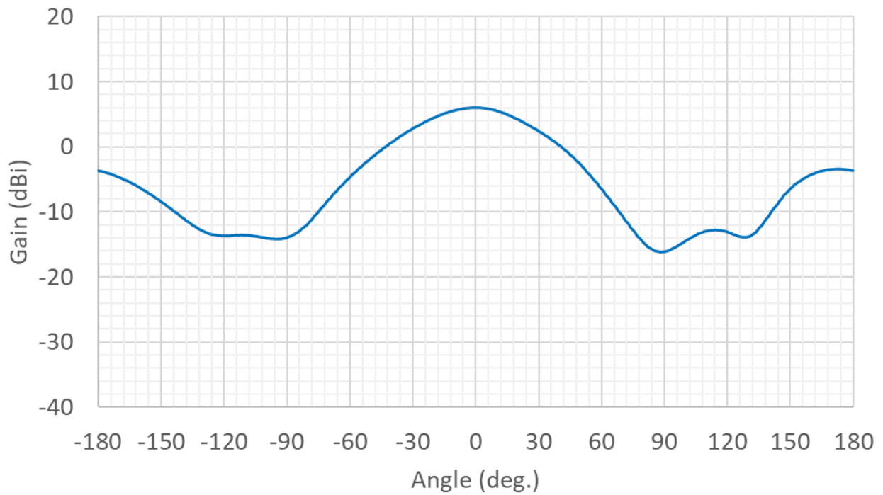
1GHz (H面)
